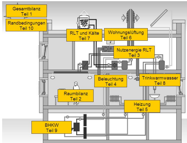
Bild 1 - Schematische Darstellung des Bilanzumfangs von DIN V 18599
